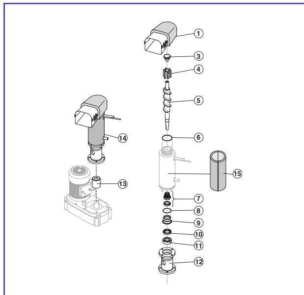
EVAPORATOR
