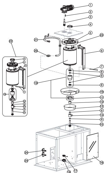
EVAPORATOR
