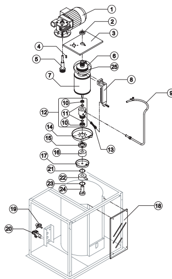
EVAPORATOR
