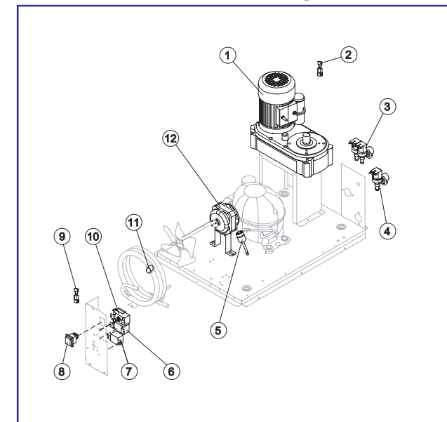
PARTI ELETTRICHE
