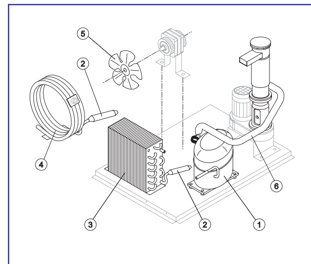
GRUPPO FRIGORIFERO
