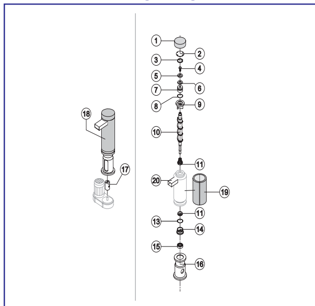
EVAPORATORE
